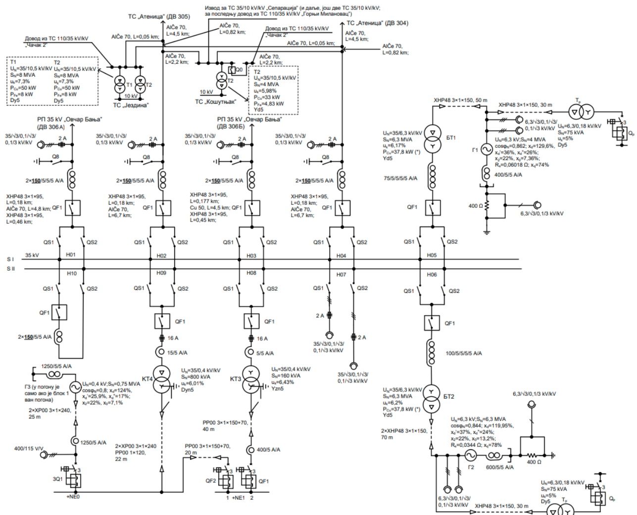
Једнополна шема ХЕ „Међувршје“
